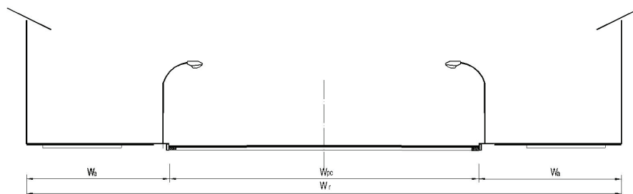
(a) 单幅路
