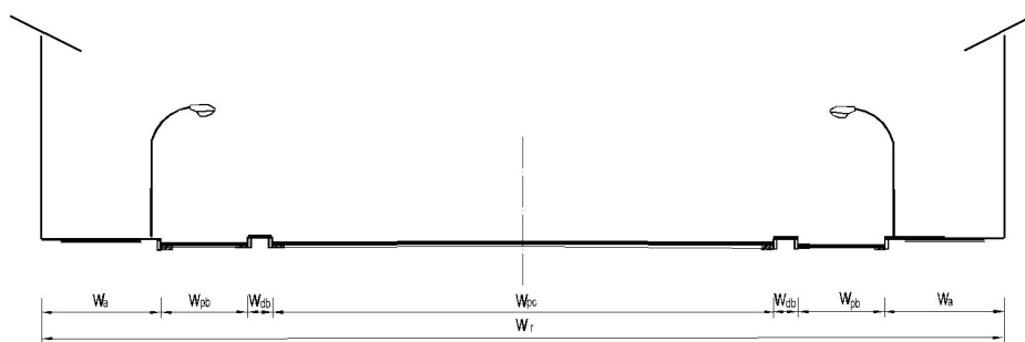
(c) 三幅路
