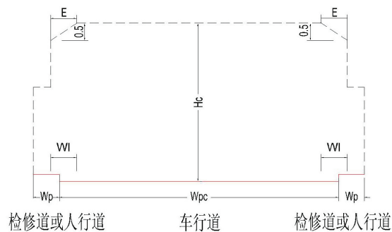
c) 隧道内
